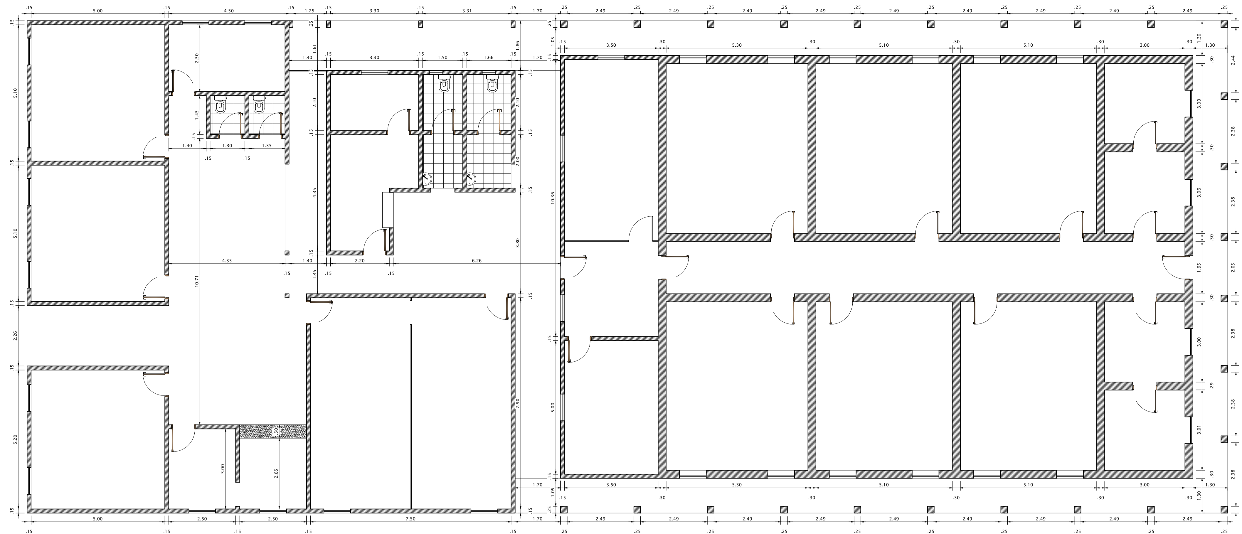
PROJETO SITUAÇÃO ATUAL ESC. 1/75
